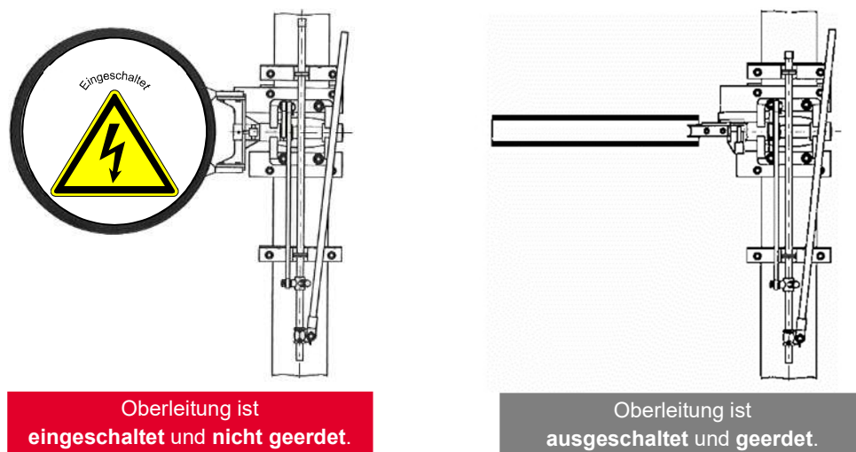
Abbildung 55 – Schaltzeiger des Ladegleisschalters – alt
